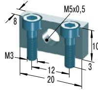
MB5SC2 *€ 13,38 Montageblok
