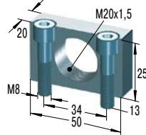
MB20SC2 *€ 16,58 Montageblok
