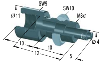
BV8A *€ 29,71 Geleidingspen
