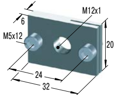
RF12 *€ 13,39 Rechthoekflens
