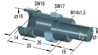
BV14SC *€ 42,86 Geleidingspen
