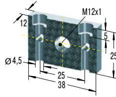
UM12 *€ 14,00 Universeelflens
