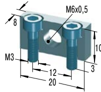
MB6SC2 *€ 12,15 Montageblok
