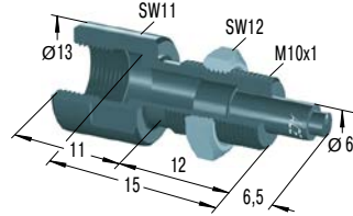
BV10 *€ 34,01 Geleidingspen
