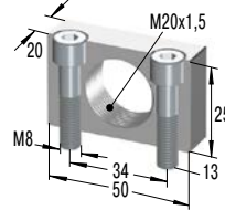
MB20SC2-V4A *€ 29,31 Montageblok
