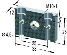
UM10 *€ 13,39 Universeelflens
