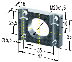
UM20 *€ 17,56 Universeelflens
