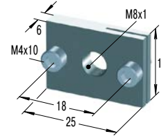
RF8 *€ 12,15 Rechthoekflens
