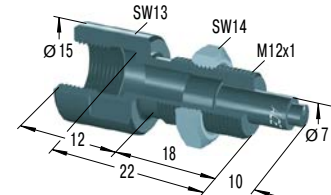
BV12SC *€ 35,97 Geleidingspen
