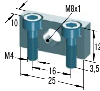
MB8SC2 *€ 12,15 Montageblok
