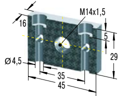
UM14 *€ 16,83 Universeelflens
