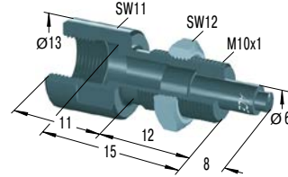
BV10SC *€ 34,01 Geleidingspen
