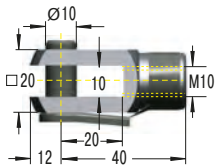
D10 Clevis Fork DIN 71752
