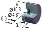
BP20 Steel/Urethane Button
