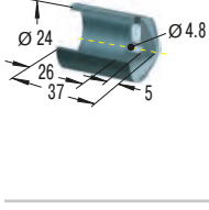
BP20 Steel/Urethane Button
