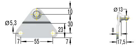
OG8-V4A Ferrure latérale à rotule
