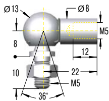
C5 Rotule radiale DIN 71802
