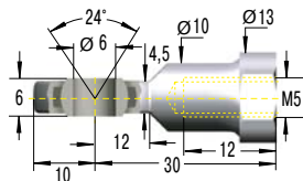
E5 Embout à rotule DIN 648
