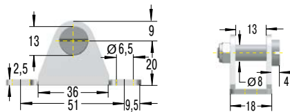
MA10-V4A Coussinet de palier
