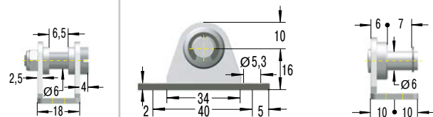
NA5 Équerre à rotule
