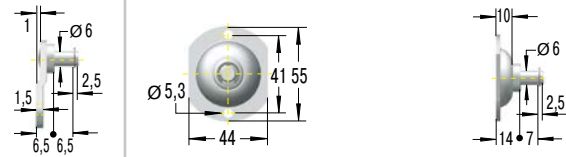
PA5 Ferrure ronde à rotule
