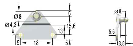
OG5 Ferrure latérale à rotule
