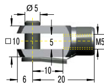
D5 Chape DIN 71752
