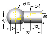
G5 Rotule sans axe DIN 71805
