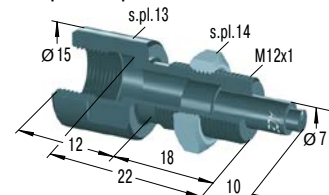
BV12SC Adaptateur pour efforts radiaux
