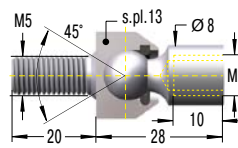
F5 Rotule axiale
