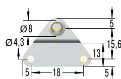
OA5 Ferrure latérale à rotule
