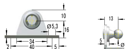
NG5 Équerre à rotule
