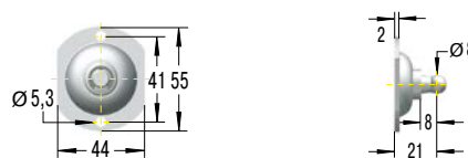
PG5 Ferrure ronde à rotule
