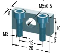
MB5SC2 Bloc de montage
