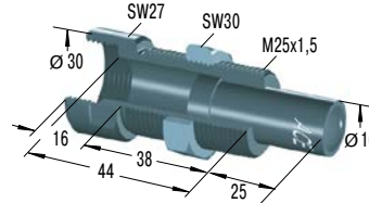
BV25SC *€ 57,80 Bolzenvorlagerung
