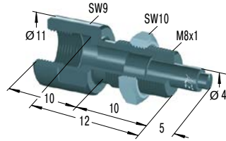
BV8A *€ 31,58 Bolzenvorlagerung
