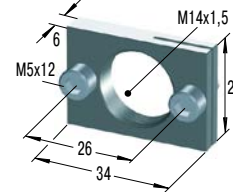
RF14 *€ 16,96 Rechteckflansch
