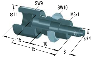
BV8 *€ 31,58 Bolzenvorlagerung
