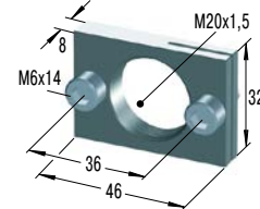
RF20 *€ 17,62 Rechteckflansch
