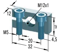
MB12 *€ 14,23 Klemmflansch
