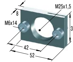
RF25 *€ 25,04 Rechteckflansch
