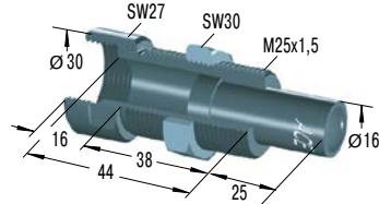
BV25 *€ 56,50 Bolzenvorlagerung
