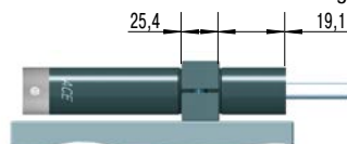
Einbaumontage für VC25...F mit Klemmblock KB... (23,8 mm für glatten Körper)
