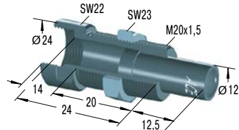
BV20 *€ 50,50 Geleidingspen
