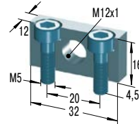
MB12SC2 *€ 14,23 Montageblok
