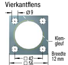
Aandraaimoment max.: 27 Nm Losbreekmoment: > 200 Nm Bevestiging met 4 schroeven
