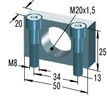
MB20SC2 *€ 17,62 Montageblok
