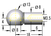
G3,5 Ball Socket DIN 71805
