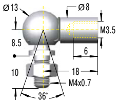
C3,5 Angle Ball Joint DIN 71802
