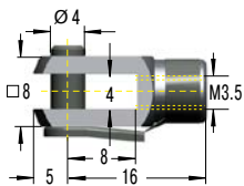
D3,5 Clevis Fork DIN 71752
